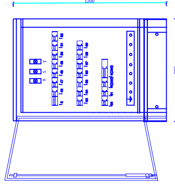
QUADRO PRIMO PIANO (Q 1P )
