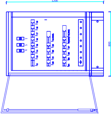
QUADRO CUCINA MENSA (Q C )
