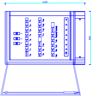
QUADRO PIANO TERRA (Q pT )
